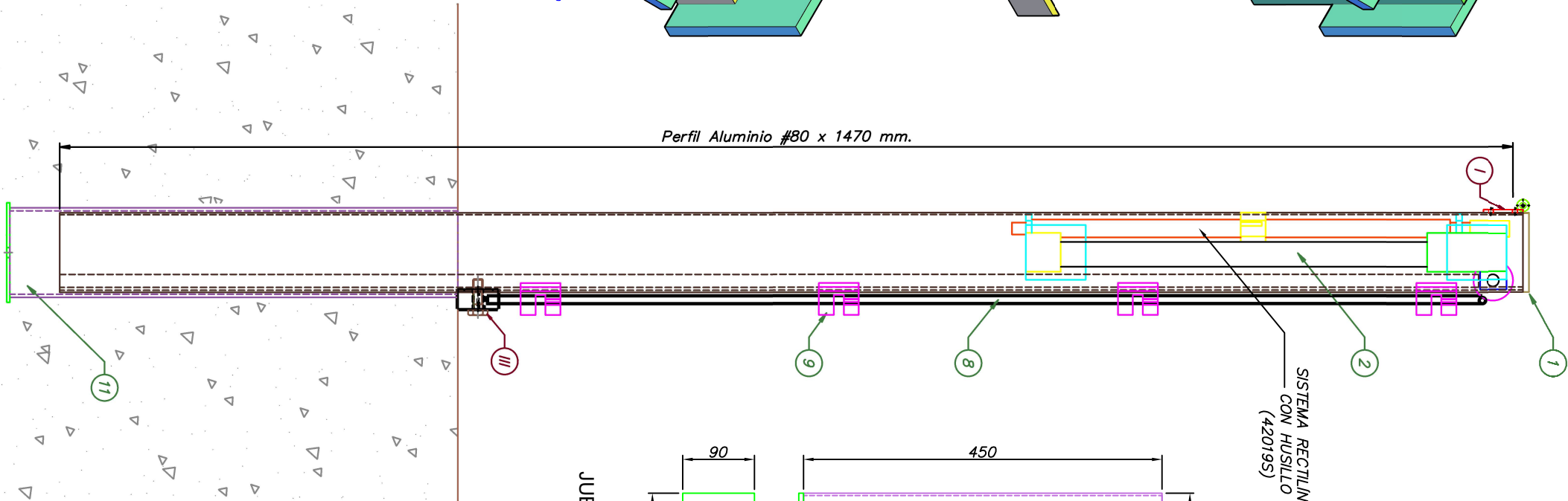
Detalle Sistema Rectilíneo de Tensado Ref: 420195 1 Unidad
