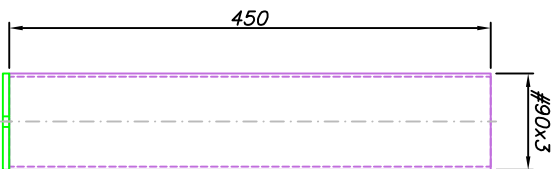
Detalle Tapa Anclaje 2 Unidades Escala 1/5
