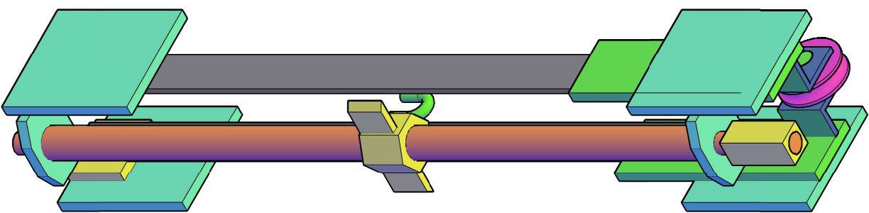
Detalle Sistema Rectilíneo de Tensado Ref: 420195 1 Unidad
