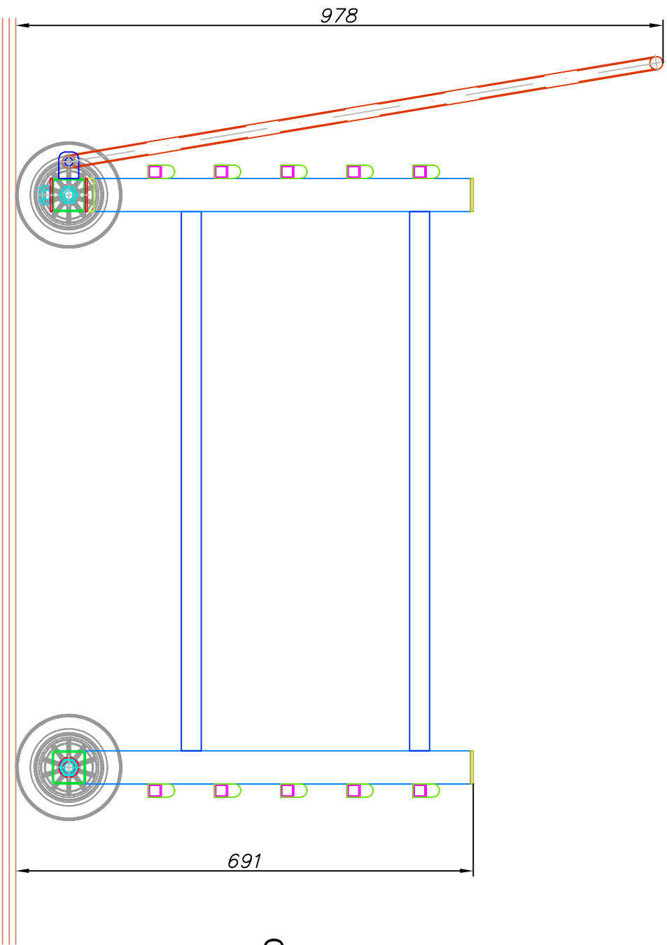
CARRO PORTA PÉRTIGAS 33420 Escala 1/8
