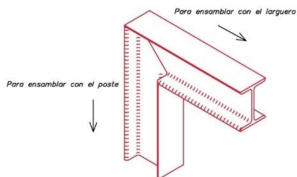
Escuadra maciza interior perfil
