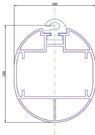
Sección transversal perfil aluminio nervado
