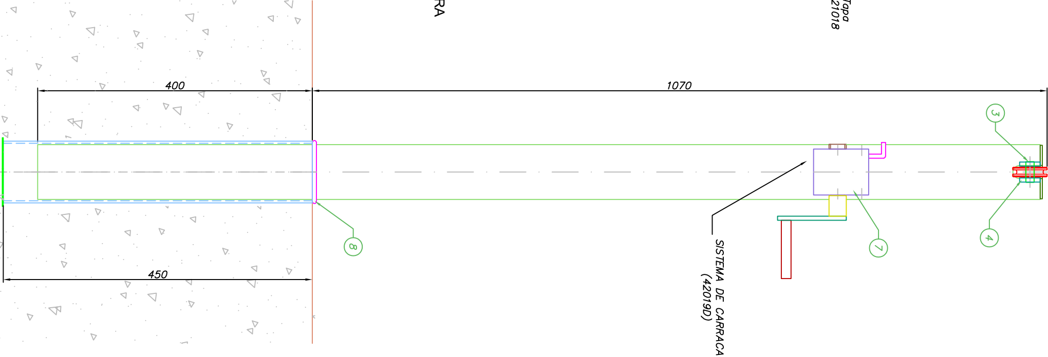
JUEGO DE ANCLAJES PARA POSTES DE Ø 80 mm. 41012 Escala 1/5
