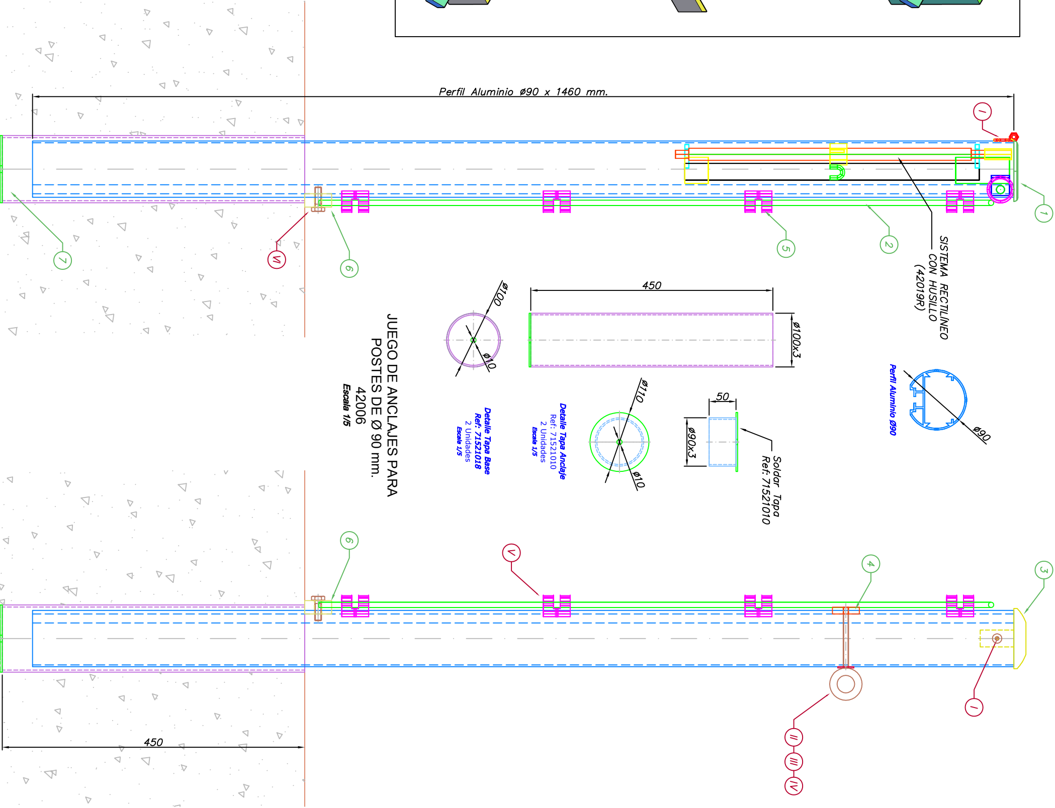
Detalle Sistema Rectilíneo de Tensado Ref: 42019R 1 Unidad
