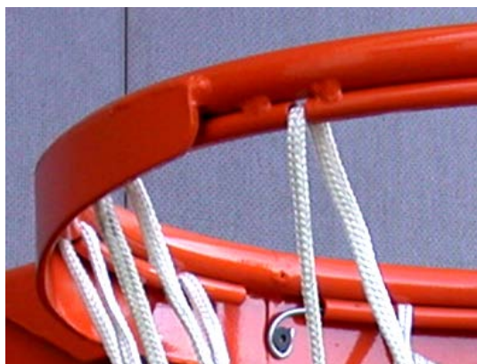
Detalle tornillo finalizador de pasador para fijación de red.
